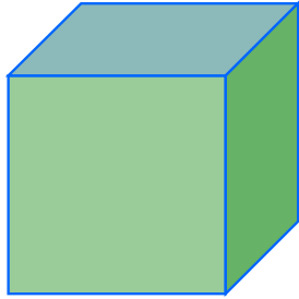
Cubo
