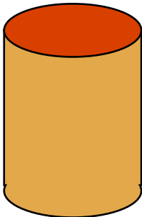
Cilindro
