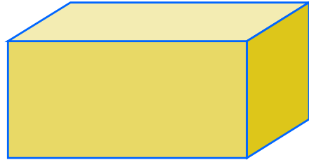
Paralelogramo
